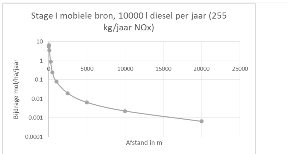
Figuur 7.1 Indicatie van de bijdrage van Stage I klasse mobiele bron met een dieselverbruik van 10.000 liter per jaar op verschillende afstanden
