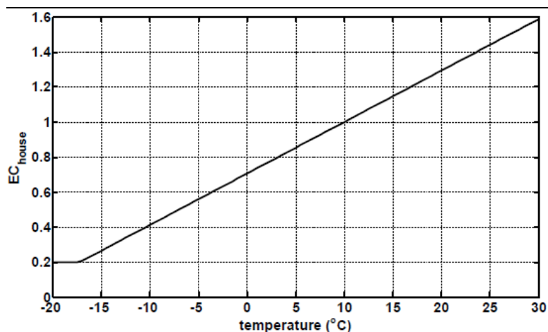
Figuur B1.4 Effect van buitentemperatuur bij profiel dierverblijven op de emissiesterkte (EC house ; 1 is de door de gebruiker opgegeven emissiesterkte)
