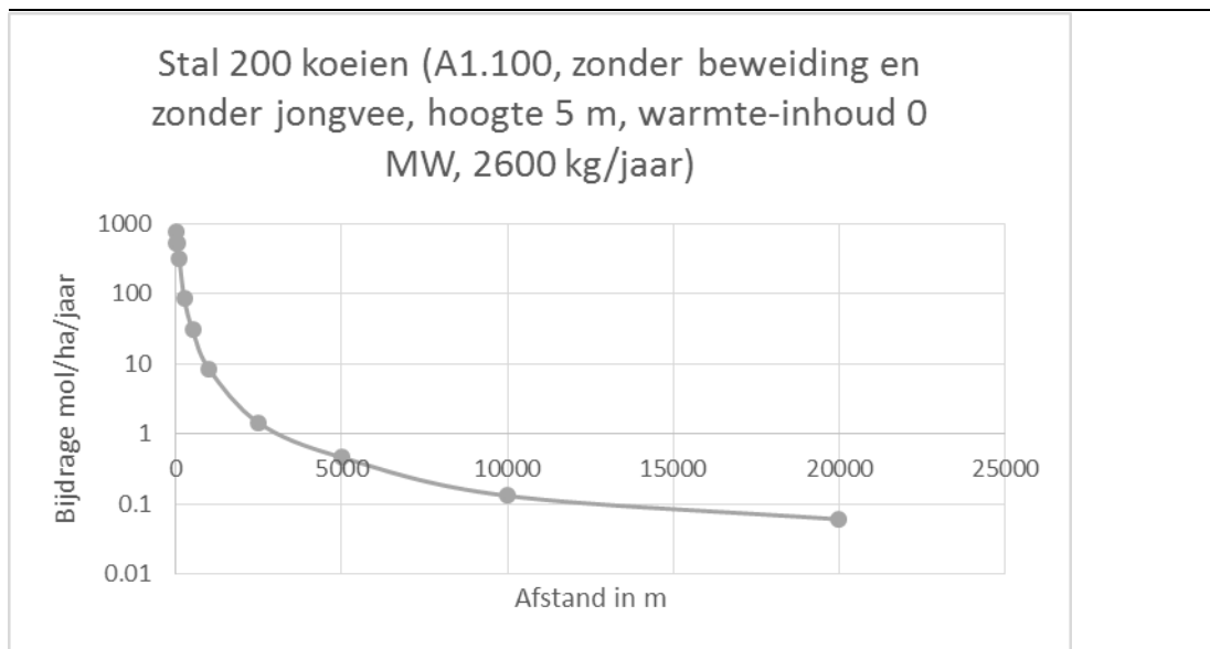
Figuur 5.4 Indicatie bijdrage stal met 200 koeien op verschillende afstanden
