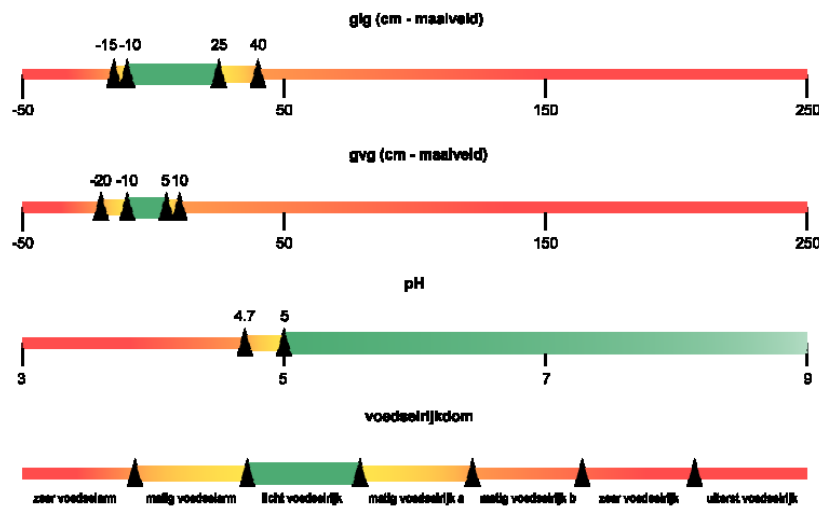
Figuur 12 Ranges voor grondwaterstand, zuurgraad en voedselrijkdom waarbij voor trilveen kenmerkende vegetaties kunnen voorkomen.
